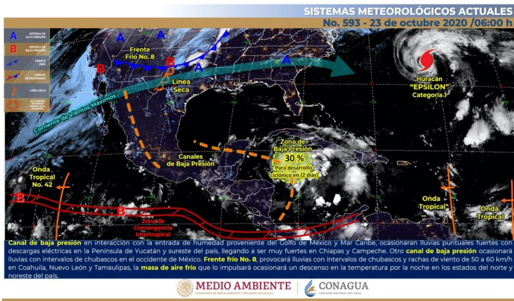
Imagen de satélite interpretada por el Servicio Meteorológico Nacional (smn.cna.gob.mx)
